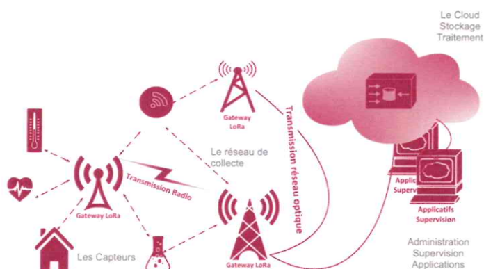
Architecture type d'un réseau LoRaWAN
